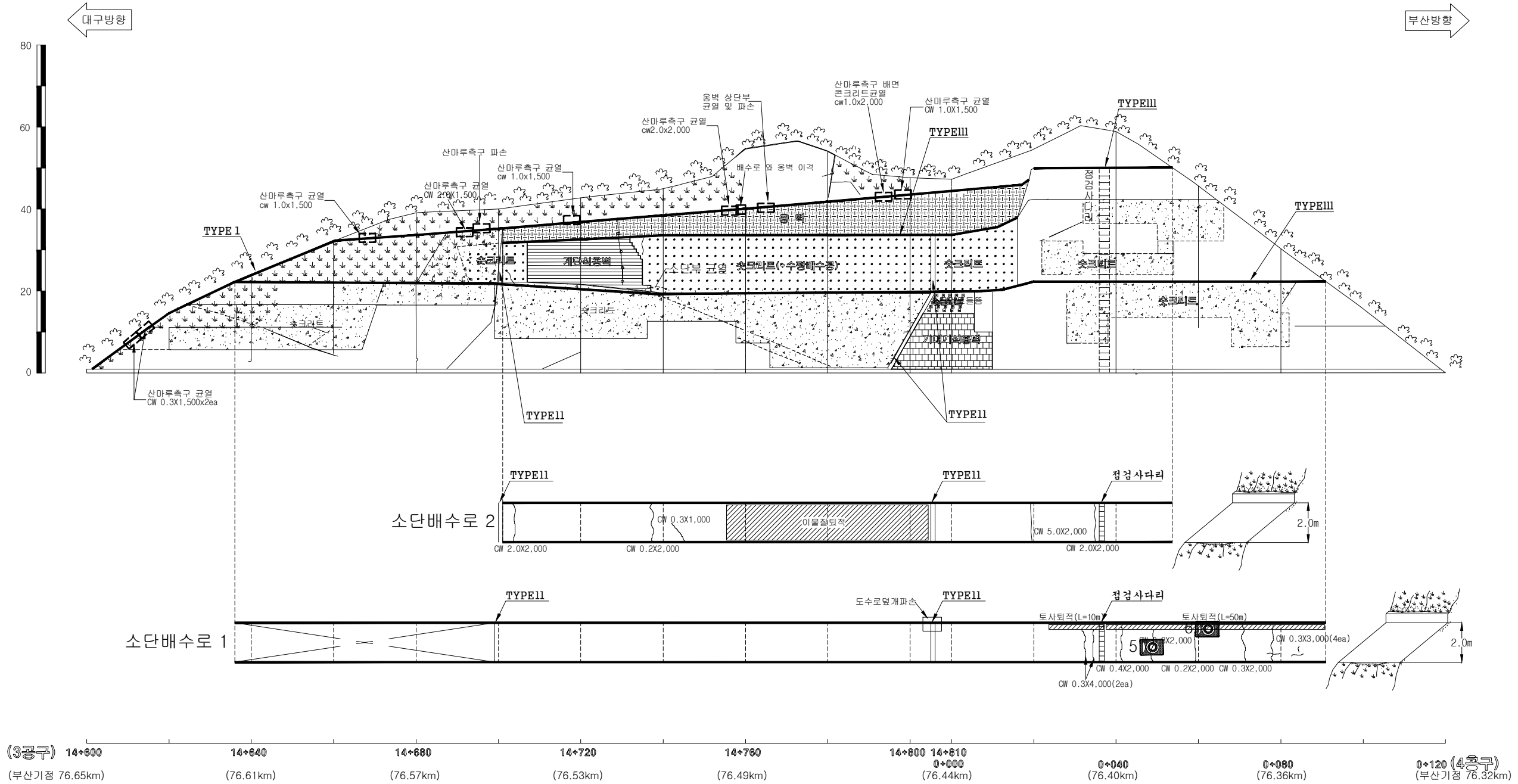
대구절토 20 / 부산기점 76.34~76.65km (3공구 STA.14+600~0+120(4공구))
